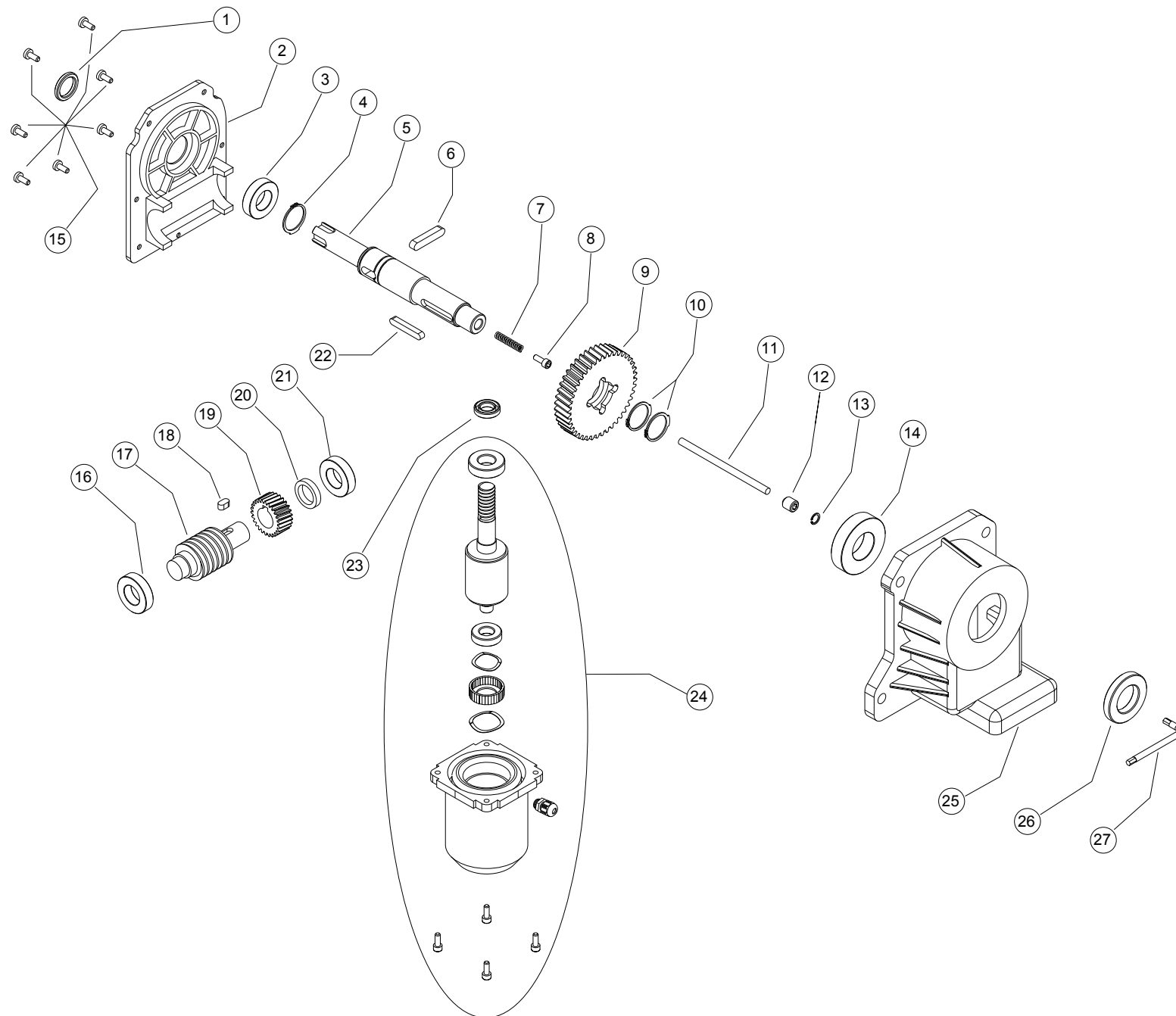
TAVOLA 2/2 MOTORIDUTTORE
