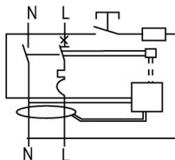
Diagrama de cableado
