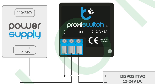
Diagrama general de conexión a dispositivo 12-24V DC:
