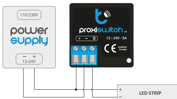
Esquema general de conexión a tiras LED 12-24V DC:
